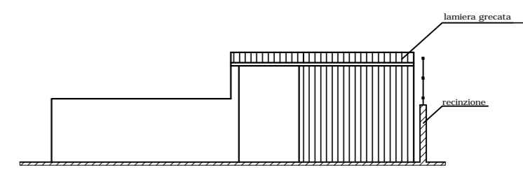
PROSPETTO D
